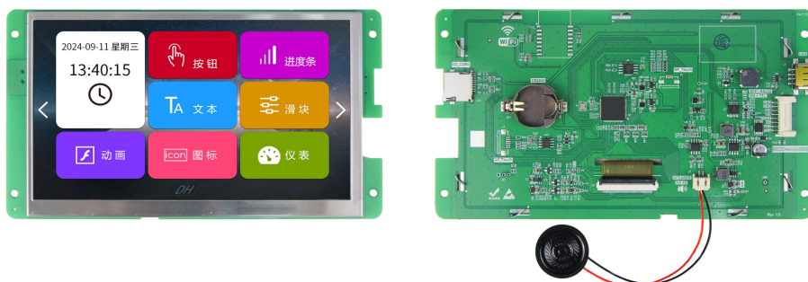
图 1-3 7.0 寸无触摸参考图
