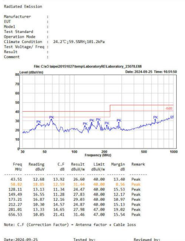
图 5-7 辐射测试垂直方向
